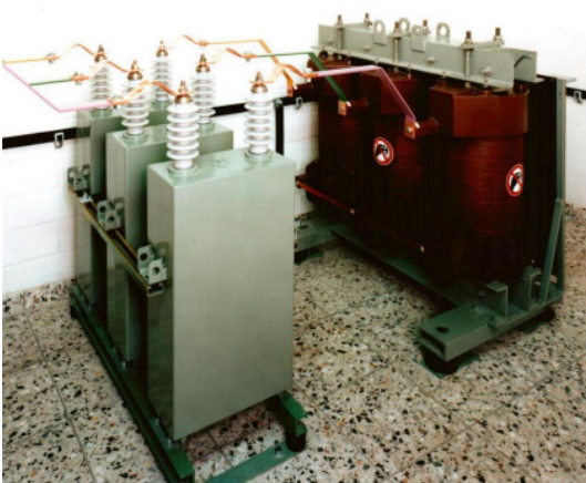
RAP für Mittelspannung (Innenraum)
