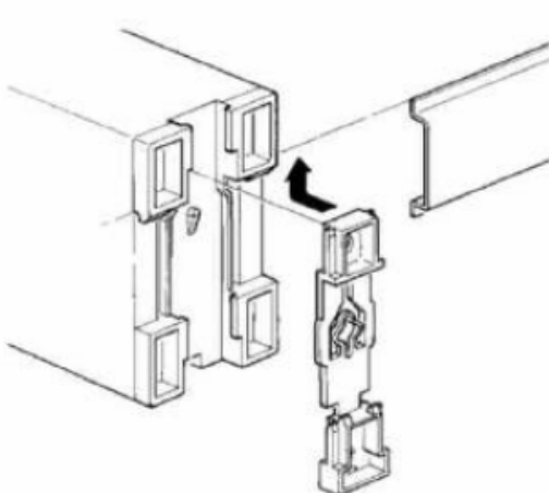
Schienenmontage
