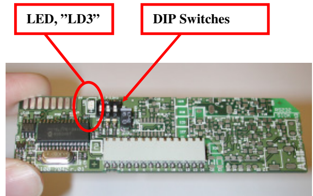
Fig. 5.1., Option board
