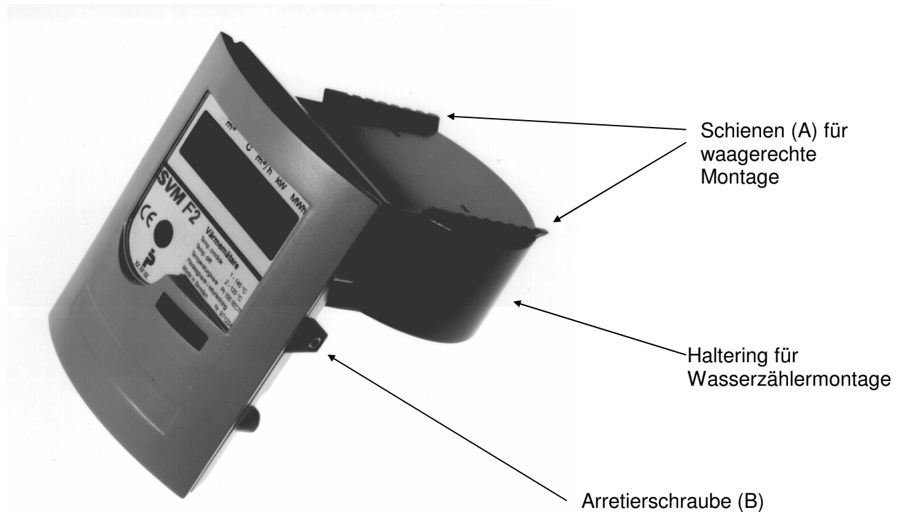
Bild 1 senkrechte Montage
